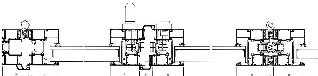
CF 77 Section de 144 mm
